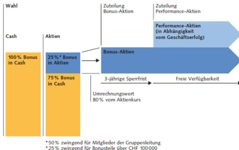
Abb. 2: Das Aktienbeteiligungsmodell
